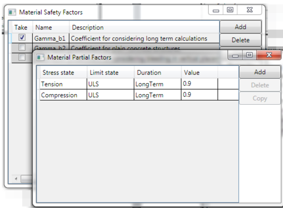
Рисунок 11-13. Коэффициенты условий работы для типа длительности и группы предельных состояний
