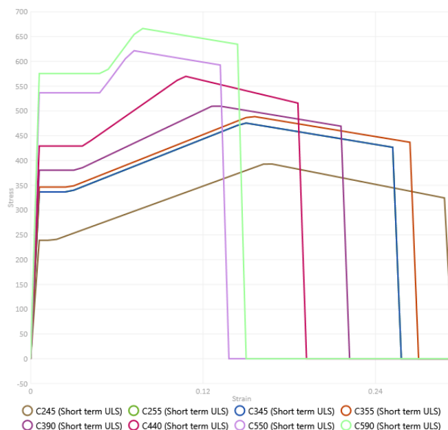
Рисунок 11-8. Обобщенная диаграмма «напряжения-деформации» по СП 16.13330.2017 (слева) и полные расчетные диаграммы в StructureHelper (справа).
