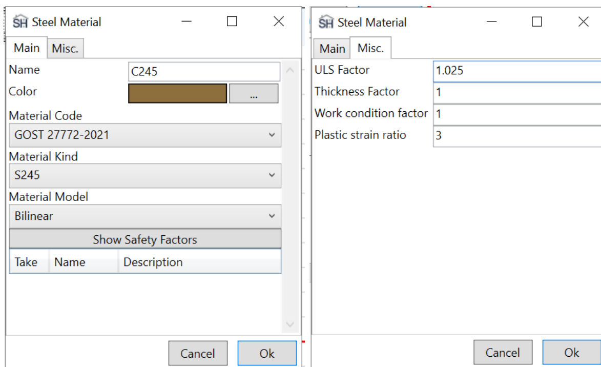
Рисунок 11-9. Свойства материала типа «Сталь» (Steel).
