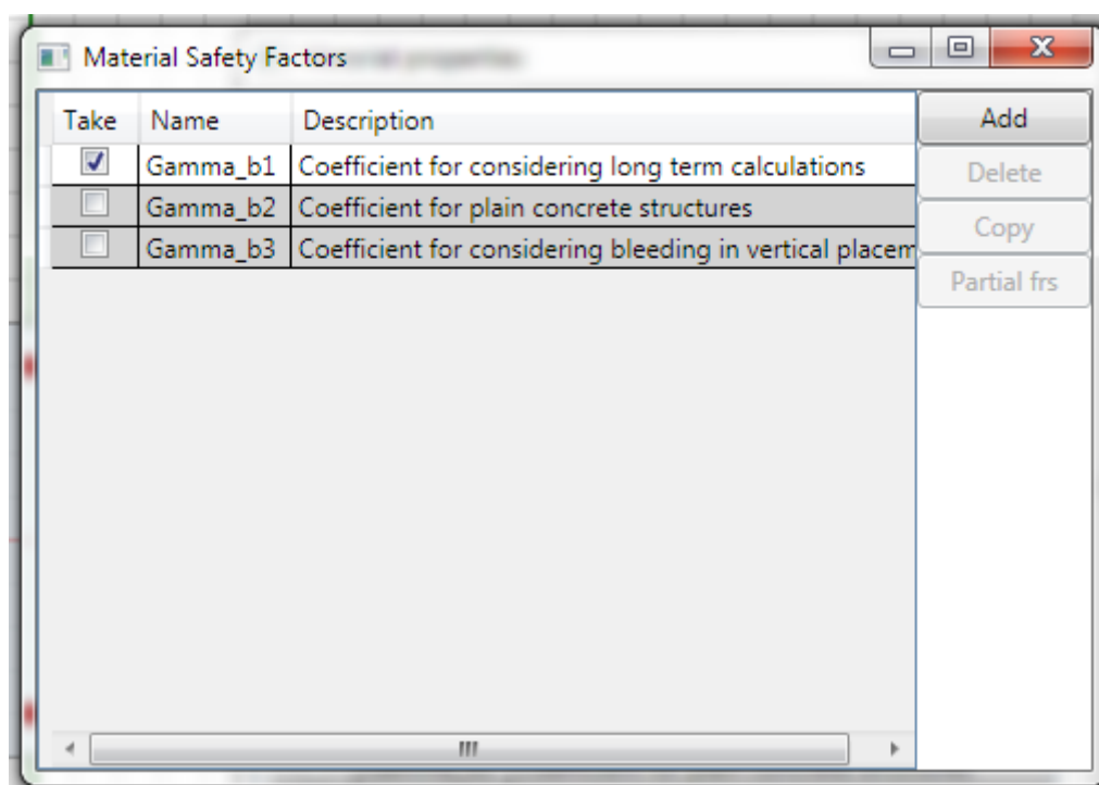
Рисунок 11-12. Коэффициенты условий работы для материалов
