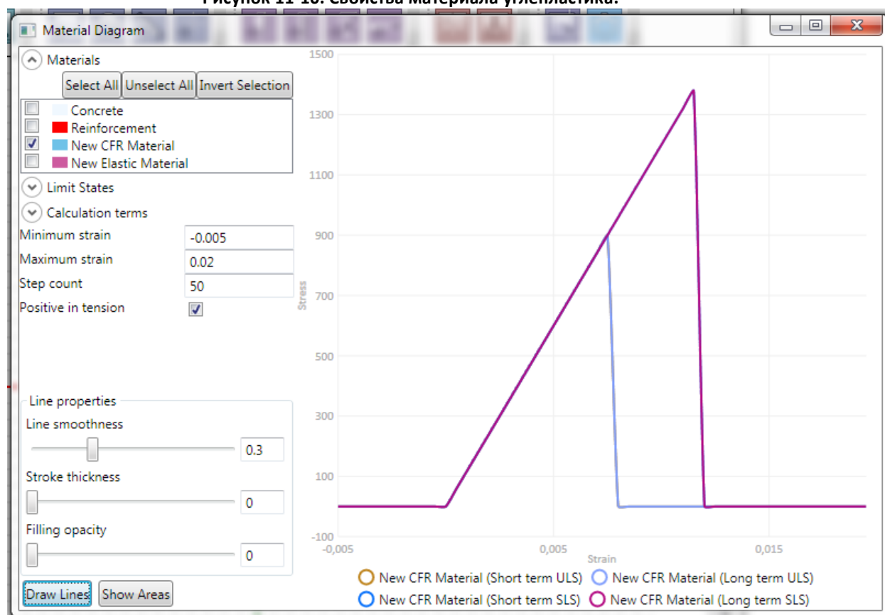
Рисунок 11-10. Свойства материала углепластика.
